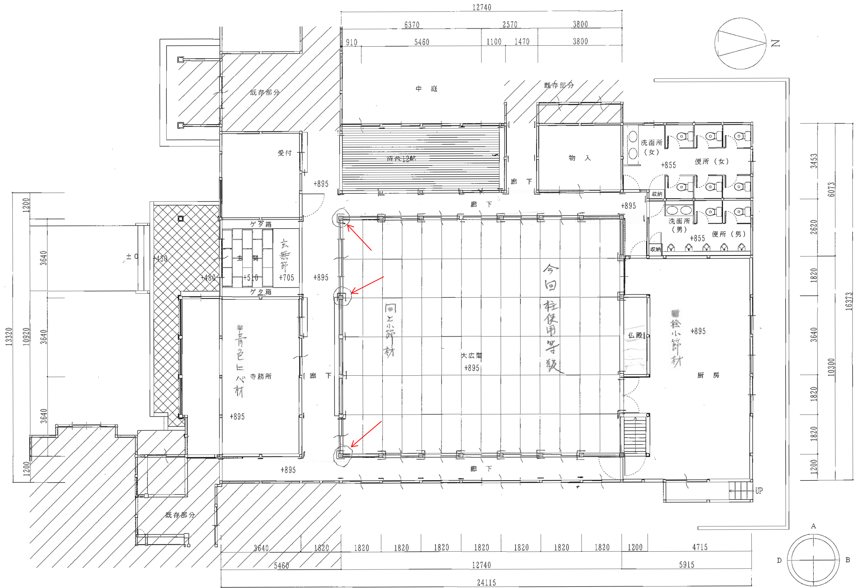
1 : 平面図 (1/100)
