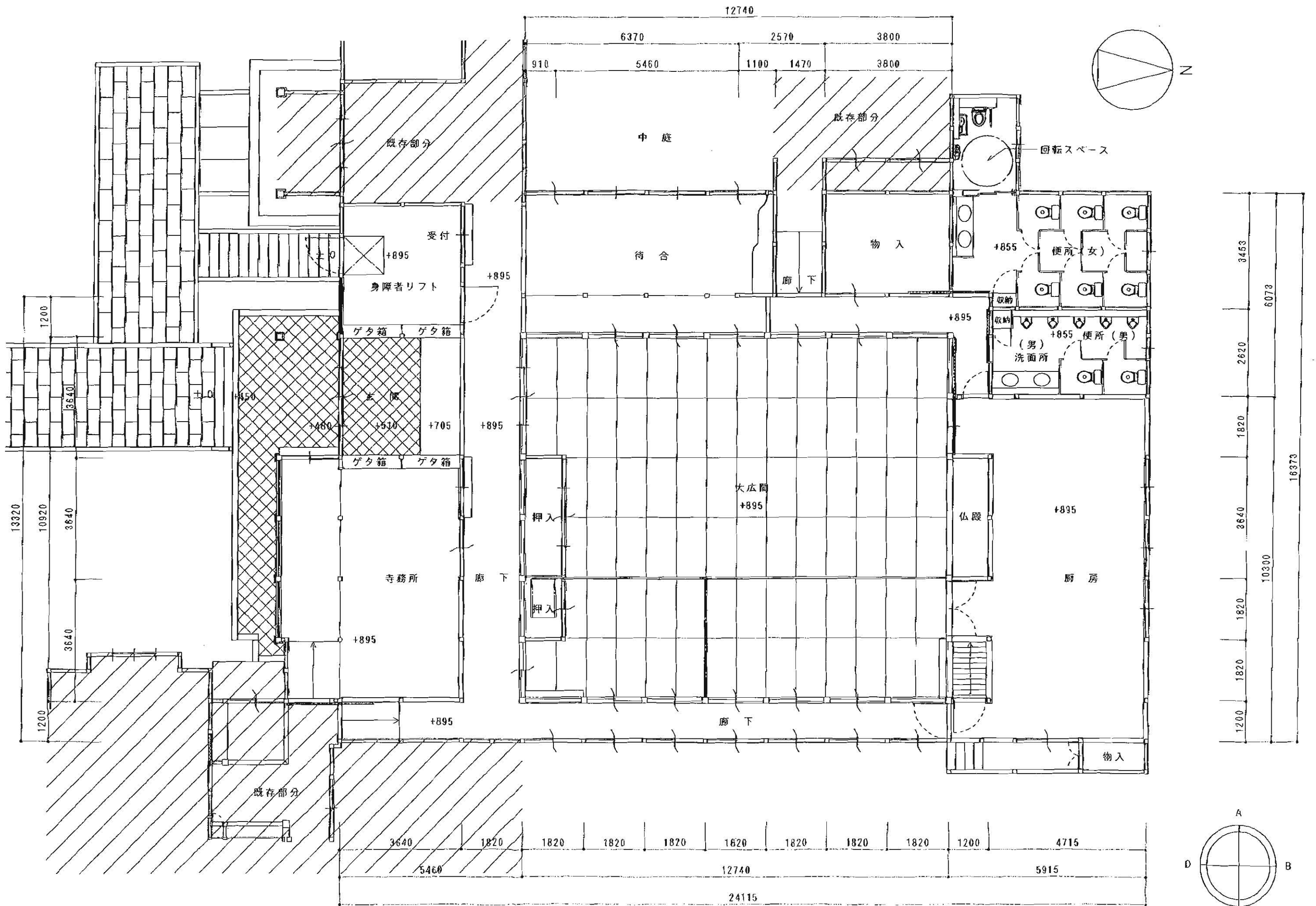
1 : 平面図 (1/100)
